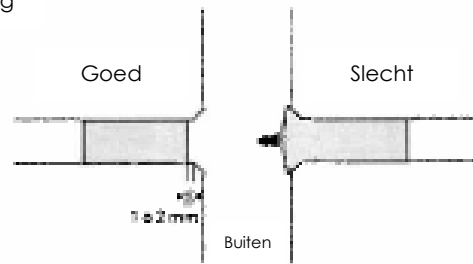
Fig. 9: Plaatsing van de dichting met inspringing
