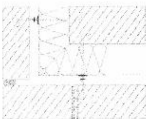
Fig. 3: Dichtingen tussen gevelelementen
