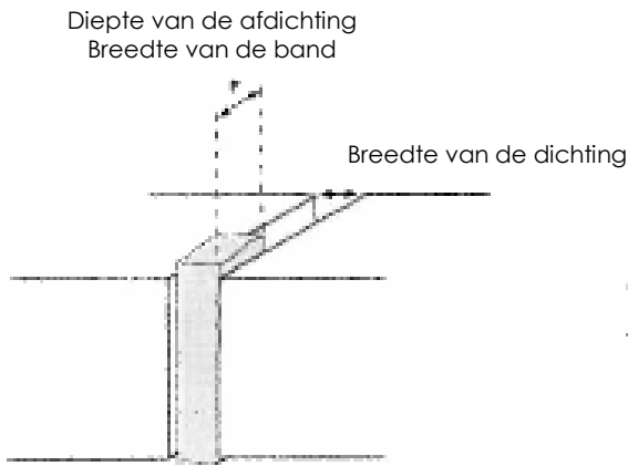
Fig. 8: Dichtingsterminologie
