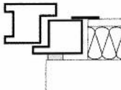
Fig. 7: Dichtingen tussen schrijnwerk en neg
