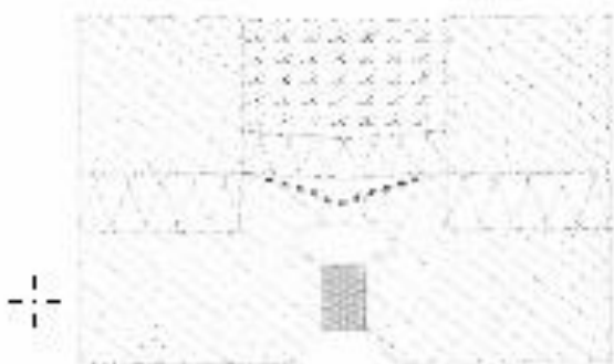
Fig. 1: Verticale dichtingen tussen zware geprefabriceerde panelen (met decompressiekamer)
