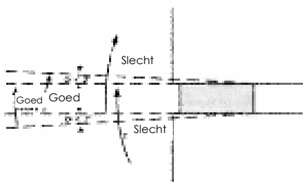
Fig. 10: Trapeziumvormige dichting
