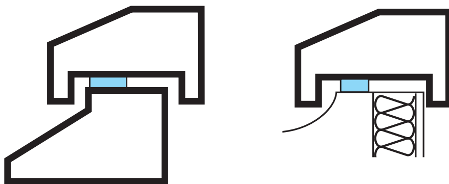
Figure 13 : exemples d'étanchéité sous pièce d'appui
