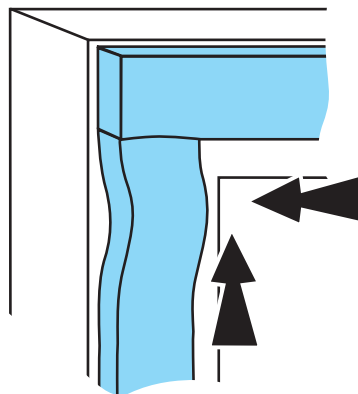
Figure 12: pose en applique et raccord à 90^\circ
