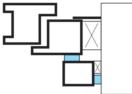
Figure 23 : pose de menuiserie sur fausse tapée
